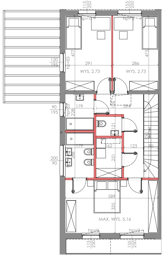
1. PIĘTRO
